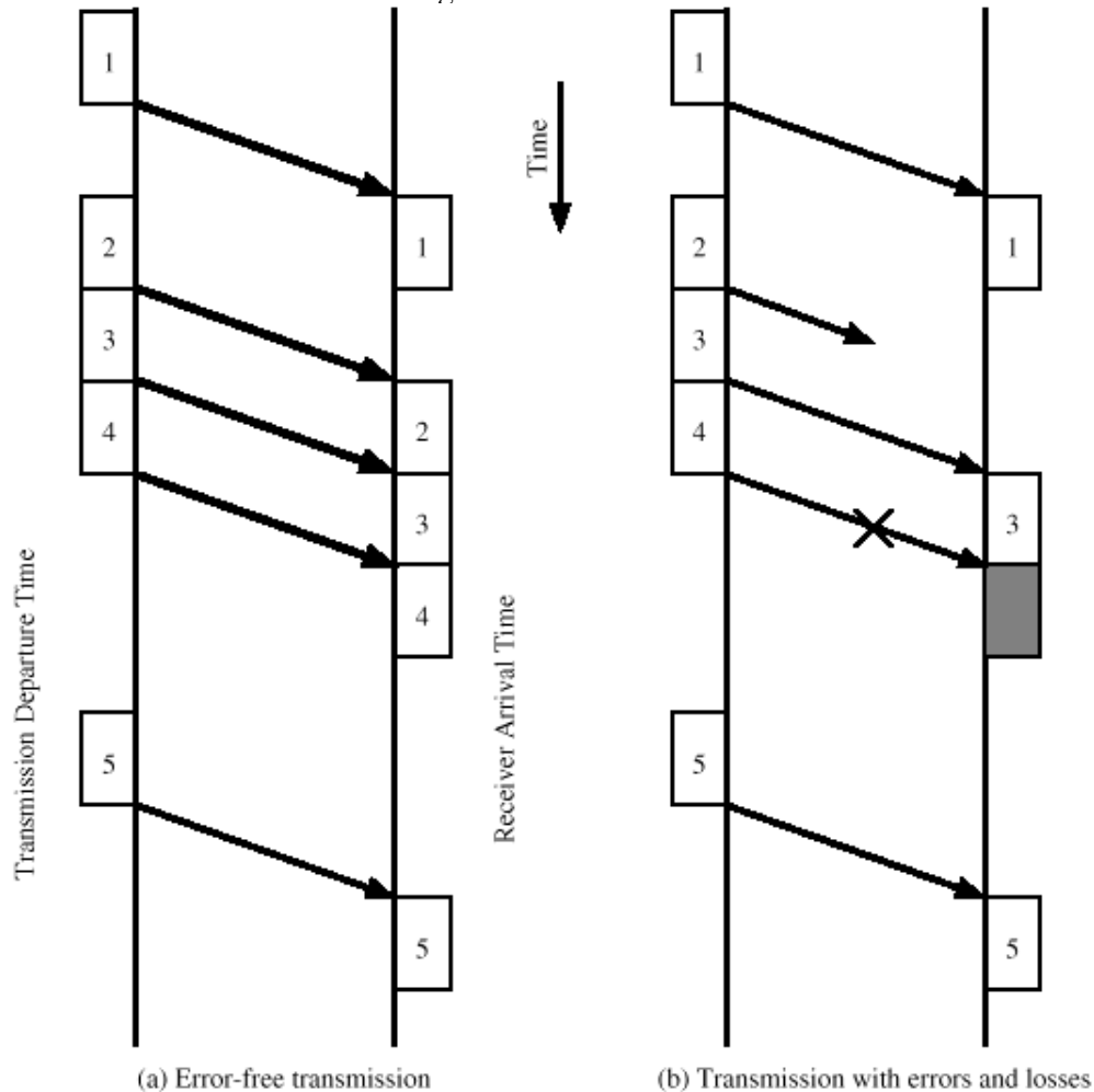
Gambar 5.4. Model dari transmisi frame
