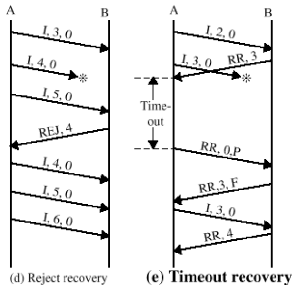
Gambar 5.15. Contoh dari operasi HDLC.
