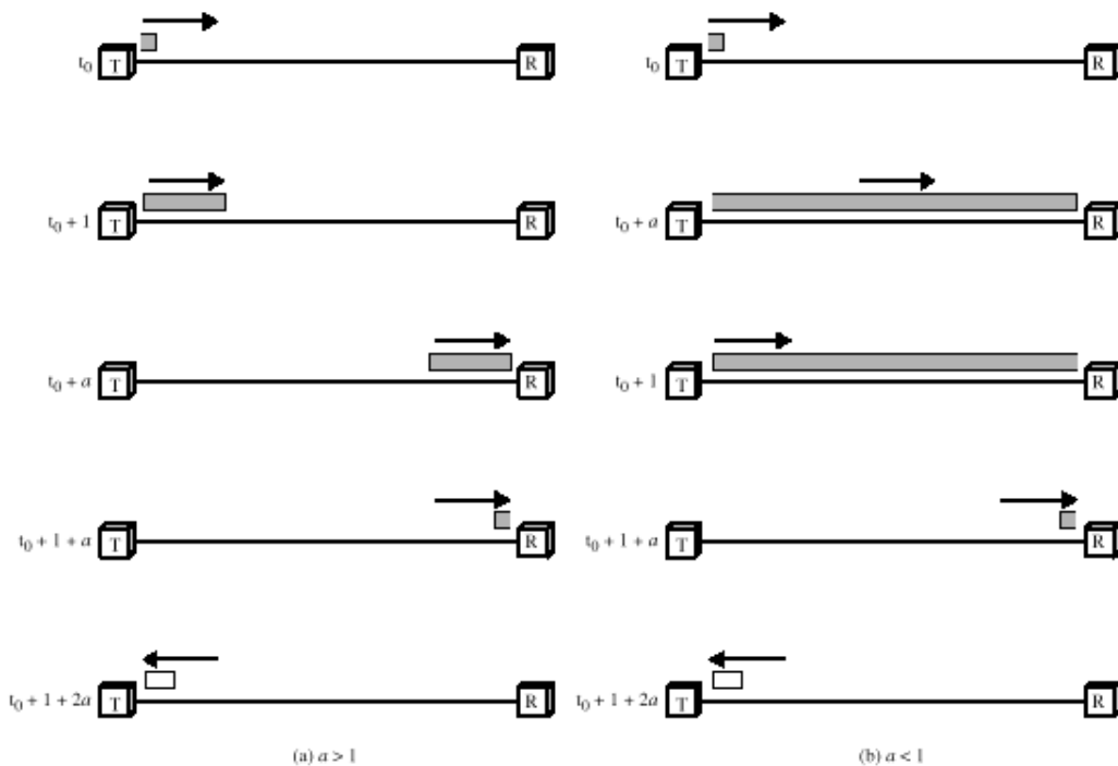
Gambar 5.5. Efek dari Utilisasi Stop and wait.
