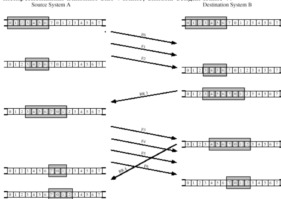
Gambar 5.7. Contoh dari protokol sliding-window.
