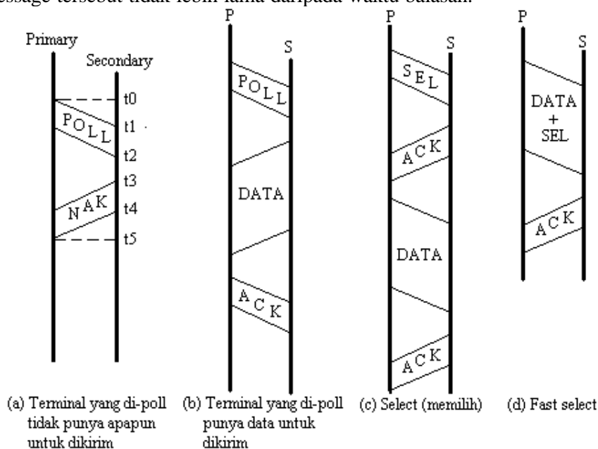
Gambar 5.3. Serangkaian poll dan select.
